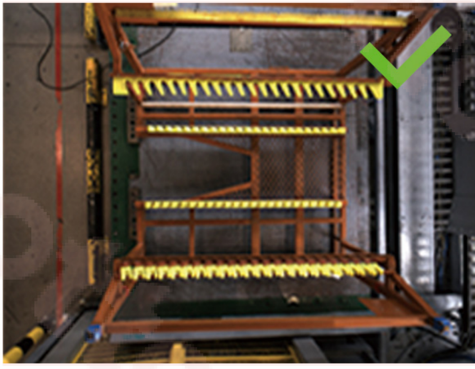
插入式料框
