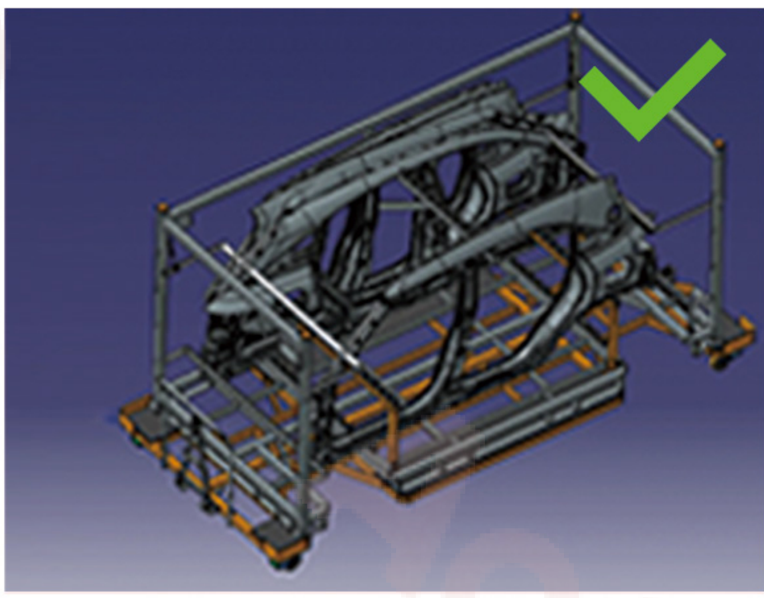
卡槽式料框
