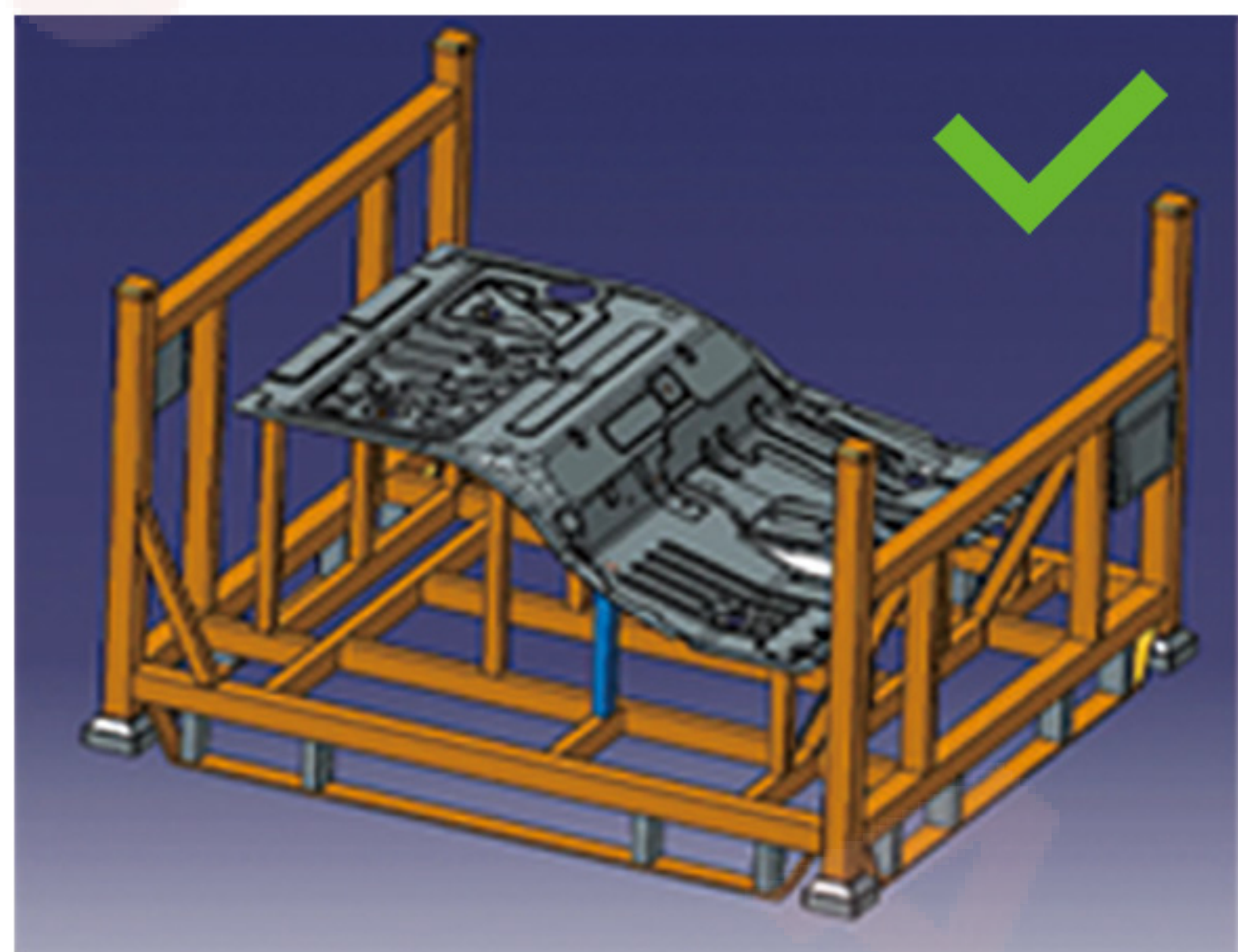
堆叠式料框
