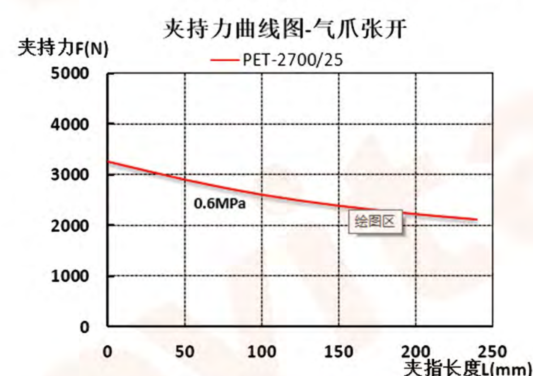
夹持力与夹指长度关系曲线
