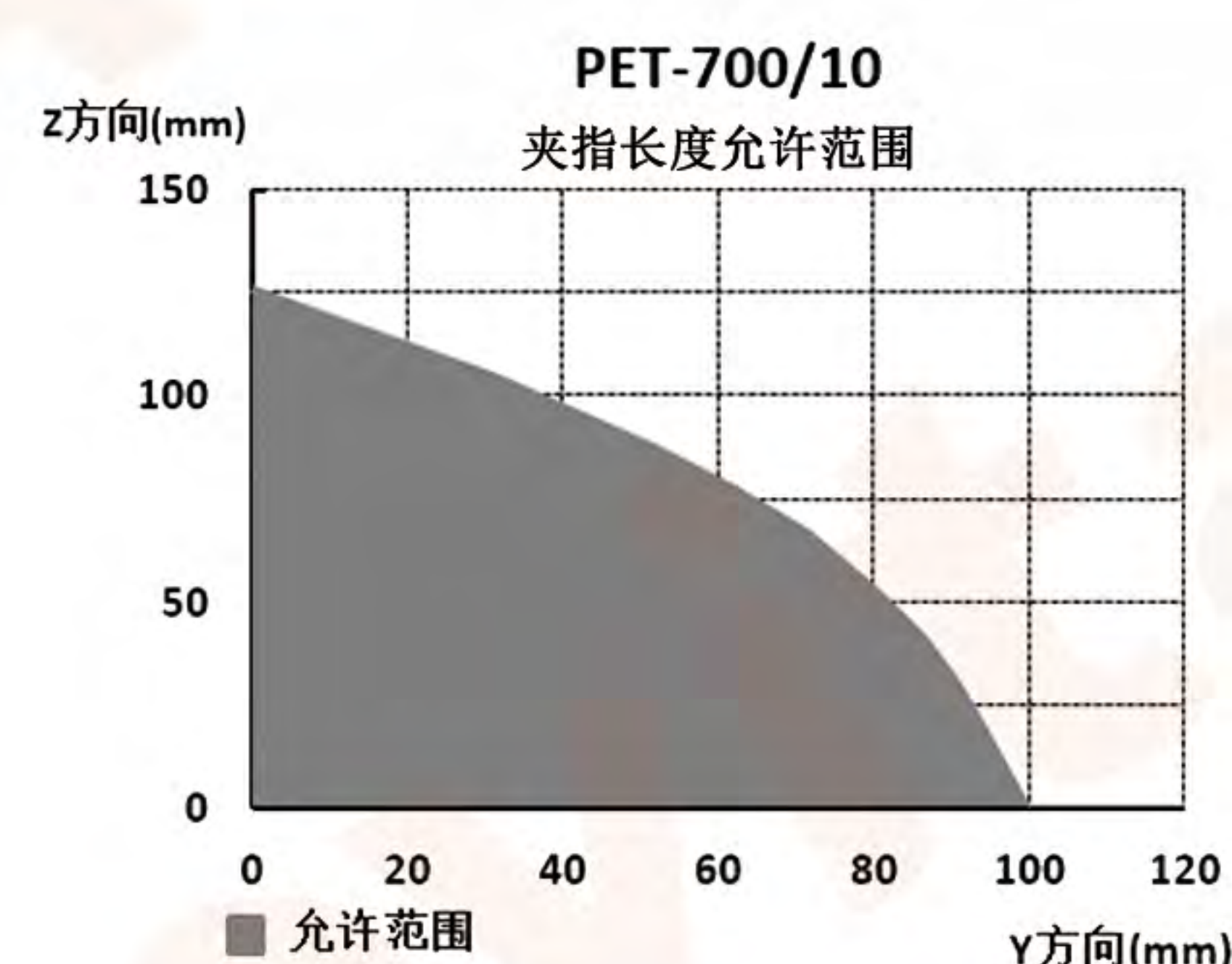
夹指长度允许范围
