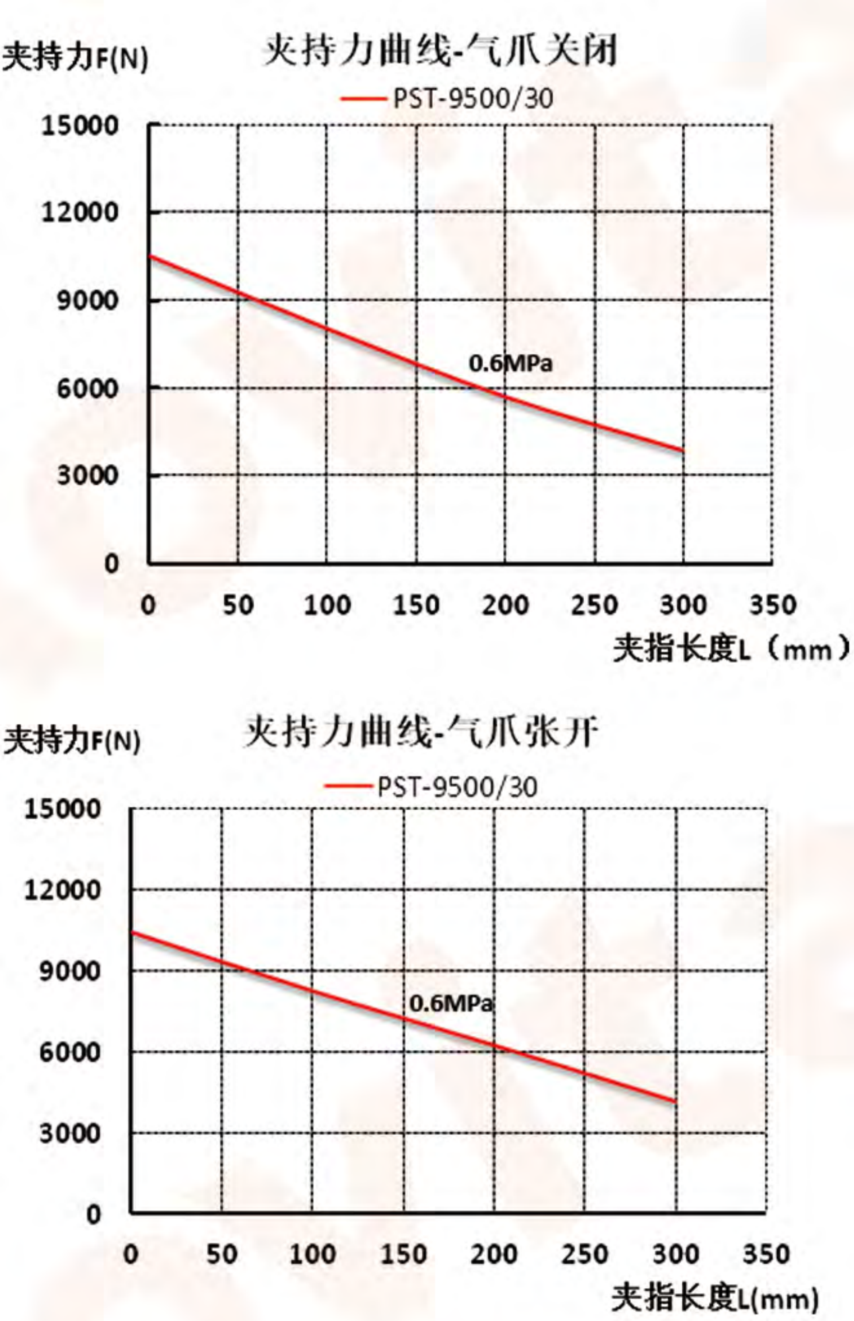
夹持力与夹指长度关系曲线
