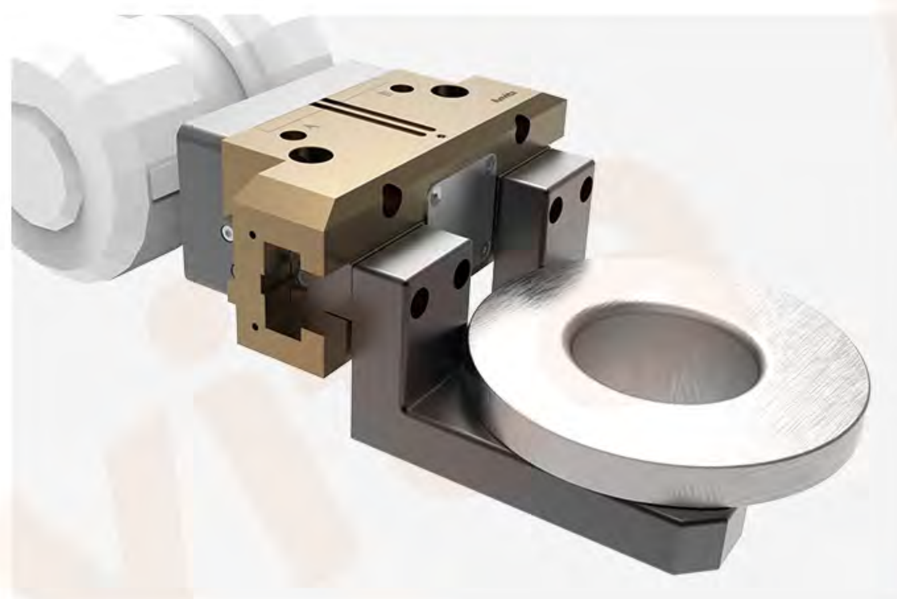
◀ 二指平行夹爪夹持轴类 / 法兰类零件
