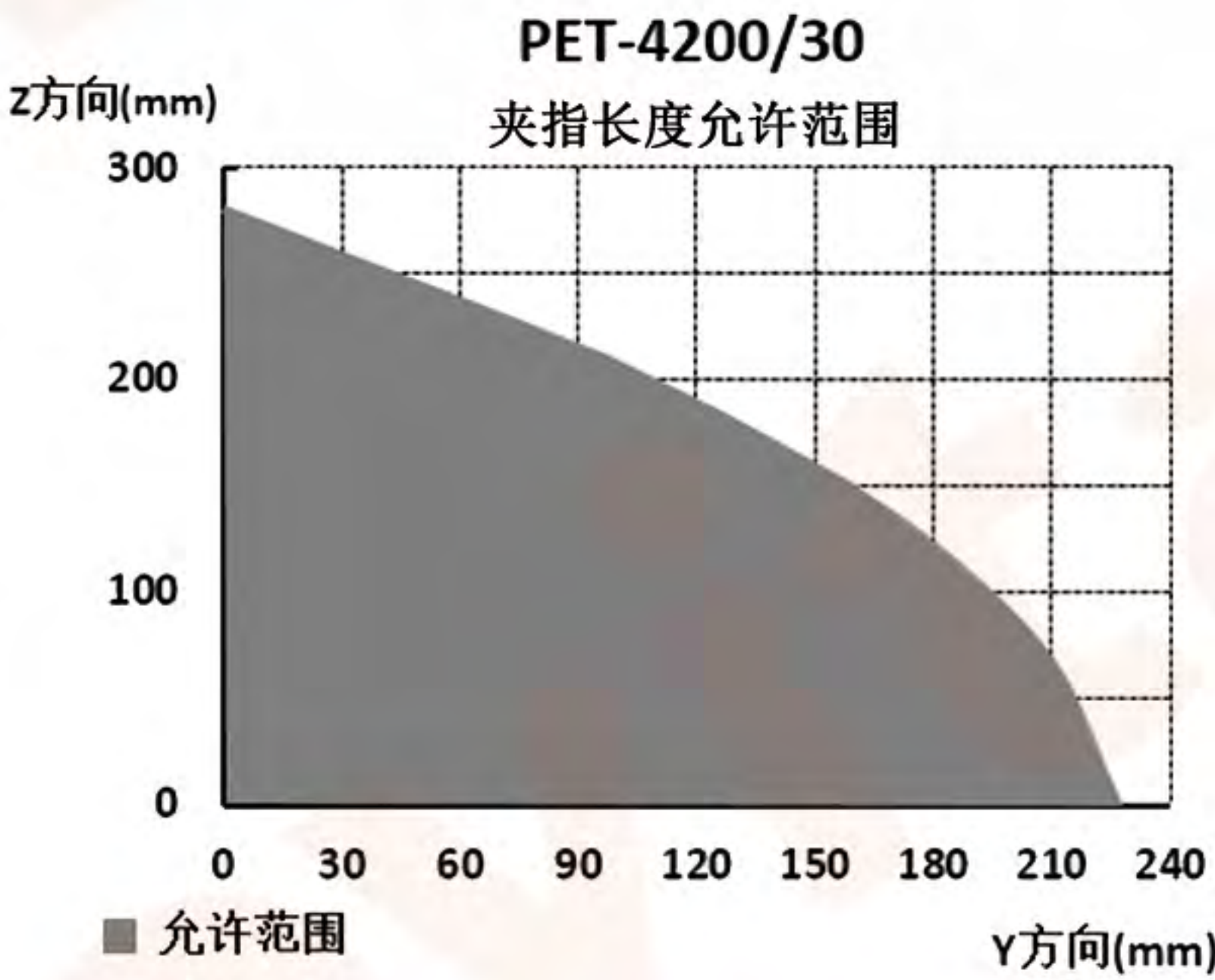
夹指长度允许范围
