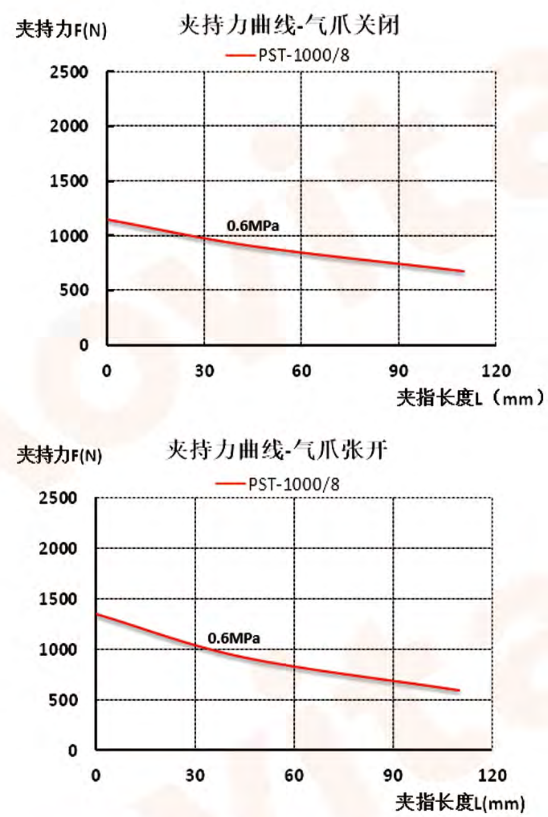
夹持力与夹指长度关系曲线
