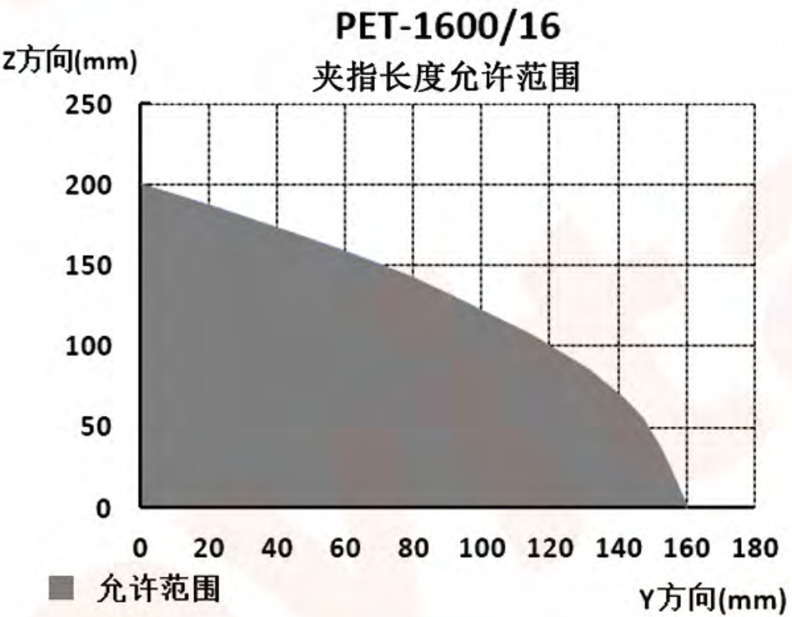
夹指长度允许范围
