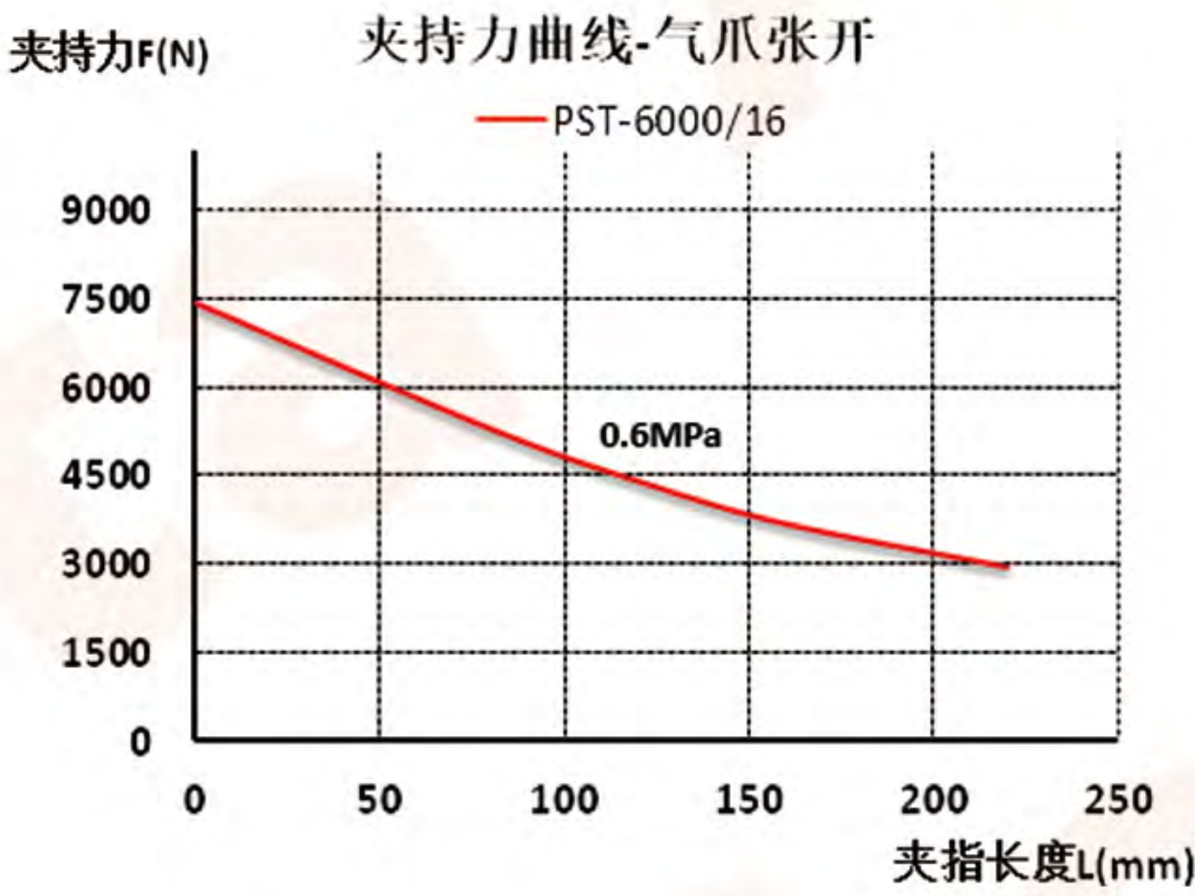
夹持力与夹指长度关系曲线
