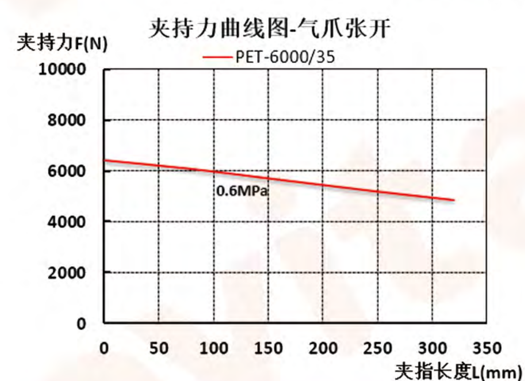
夹持力与夹指长度关系曲线
