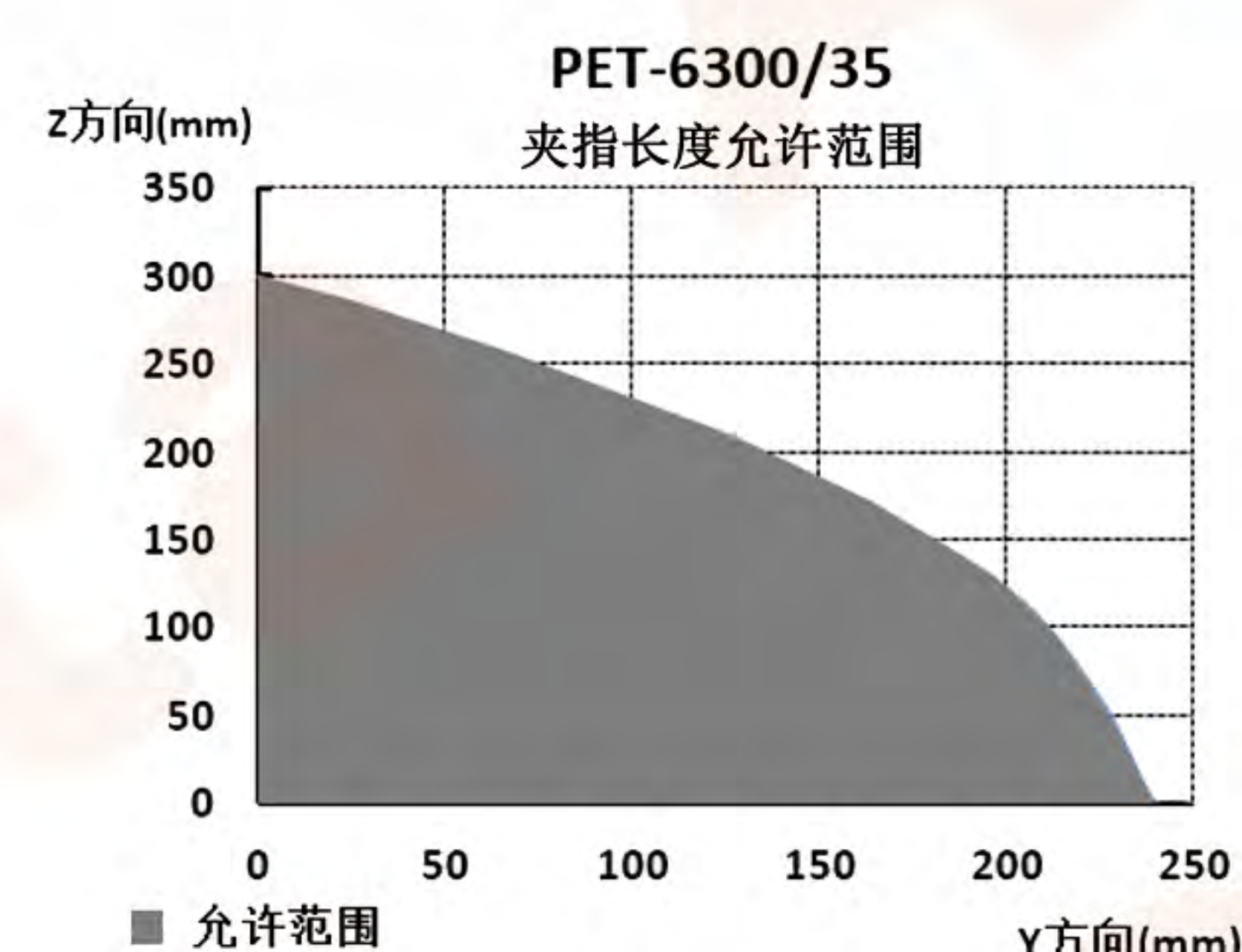
夹指长度允许范围
